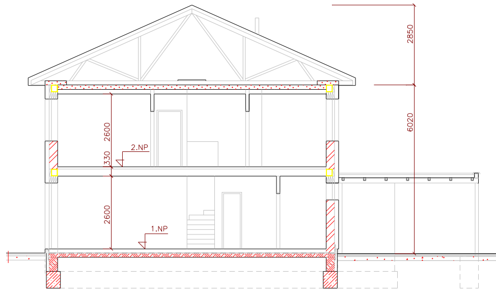
ŘEZ A-A
