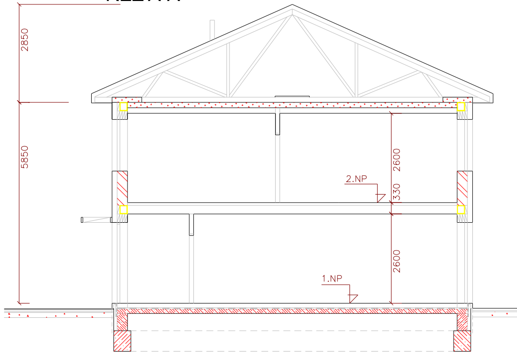
REZ A-A
